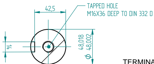
Przekrój A-A 1:2
